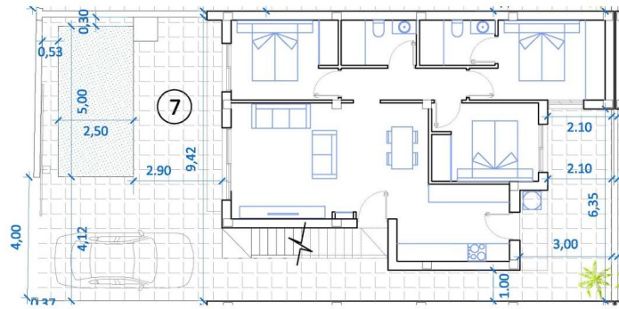
PARCELA 7: 185,30 m2.
