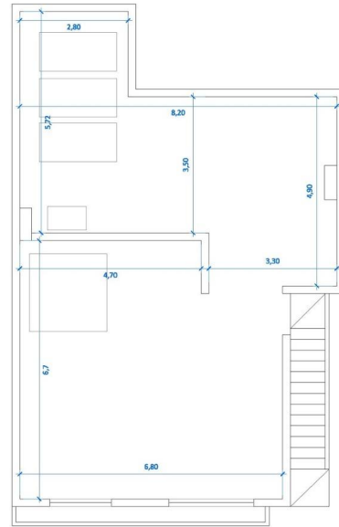
Solarium (92,20 m2)
