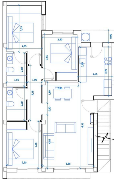
PLANTA BAJA (91,10 m2)
