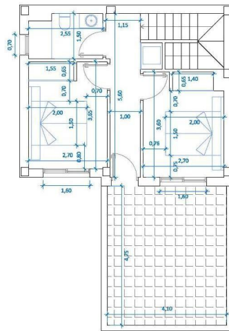
PLANTA PRIMERA
