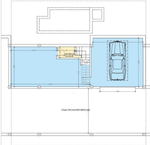
PLANTA SOTANO
