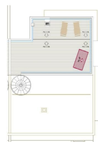
PLANTA CUBIERTA
