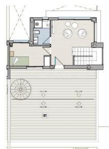
PLANTA PRIMERA
